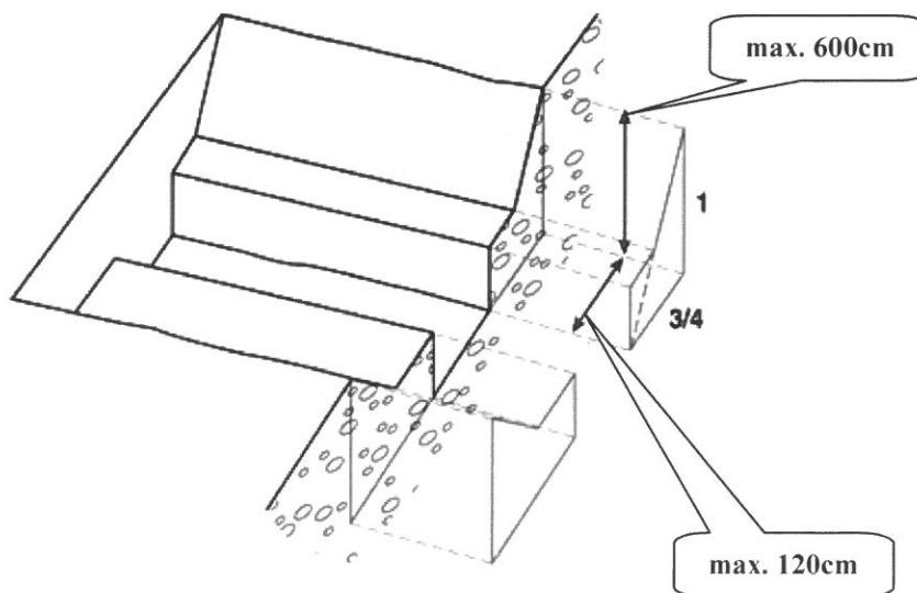
Obrázek 2, Technika svahování [7]
