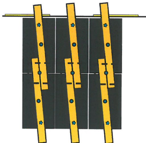
Obrázek 30, Tesařské napojení bednicích desek pod úhlem
