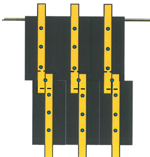
Obrázek 29, Napojení bednicích desek do hloubky výkopu 5m
