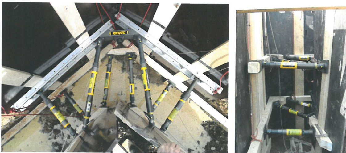
Obrázek 59, Konečná fáze stabilizace rohového výkopu [5]
