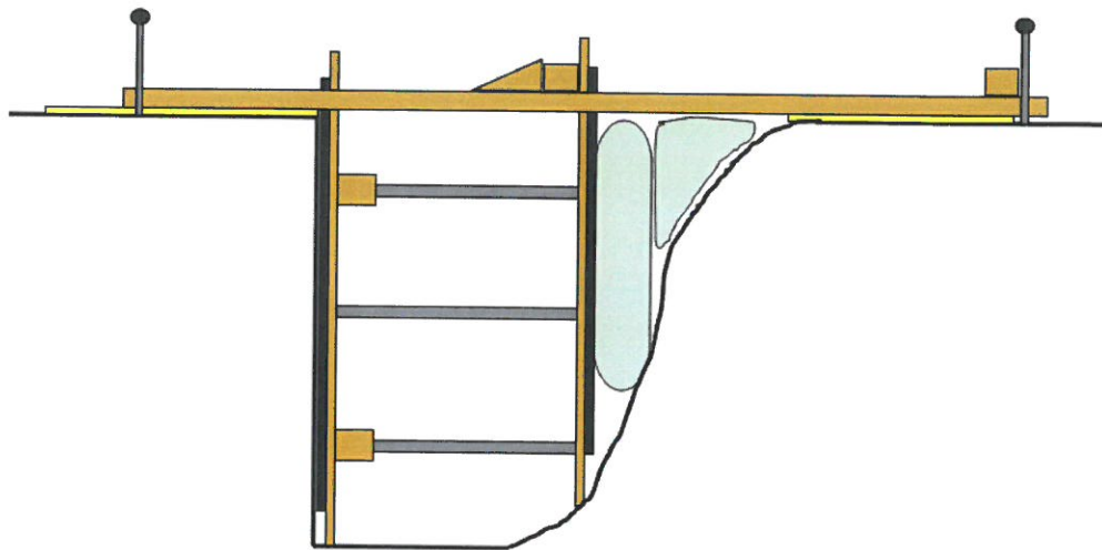
Obrázek 49, Řešení stabilizace výkopu tvaru "T" v řezu
