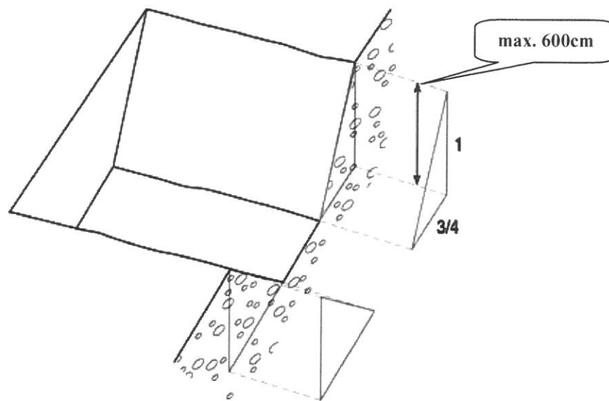
Obrázek 3, Technika svahování, šikmá plocha bez teras [7]
